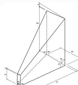
Winkelaufleger- und Einlagedetails
