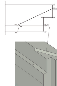
Winkelaufleger- und Einlagedetails
