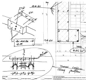
Skizze Attikasturz
